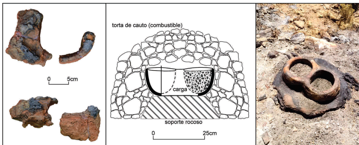
Figura 8 Horno de cauto. Fotografías de fragmentos remontados mostrando uno de los receptáculos. Corte del mismo mostrando la capa de cauto, y fotografía de un modelo experimental después de haber sido cocido.
