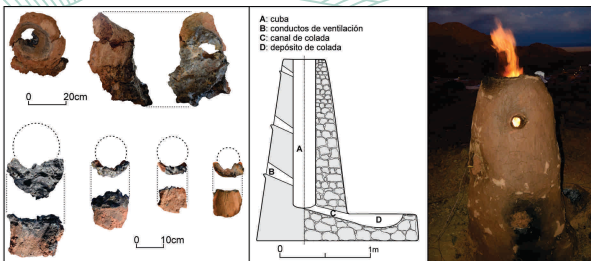
Figura 5 Horno de cuba grande. Fotografías de los fragmentos de conductos de ventilación, corte del horno y modelo experimental en funcionamiento.
