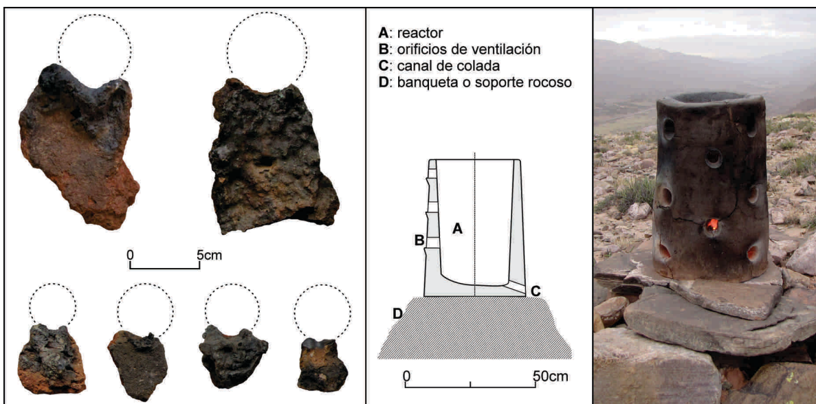
Figura 6 Wayra en arcilla. Fotografías de fragmentos con orificios de ventilación, corte del horno y modelo experimental en fin de ciclo de fundición.
