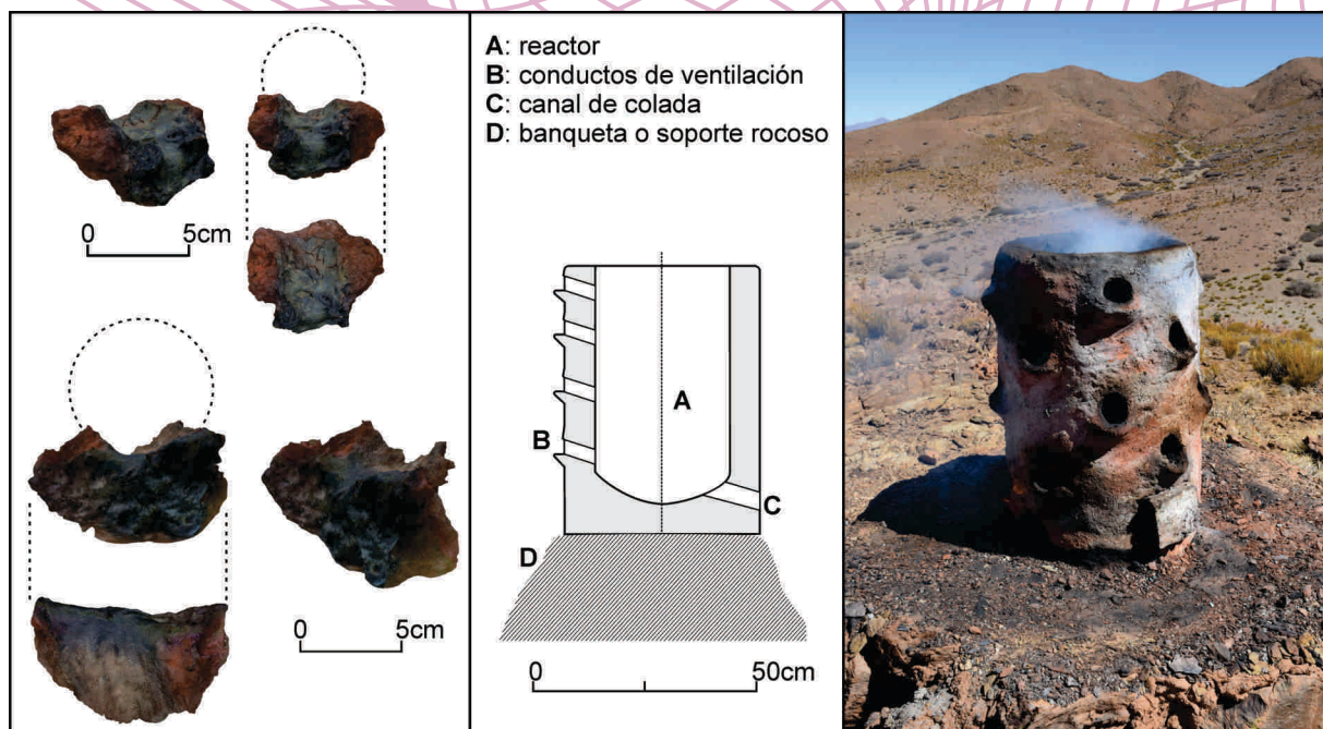
Figura 7 Wayra de paredes gruesas. Fotografías de los orificios de ventilación, corte del horno y modelo experimental en funcionamiento.
