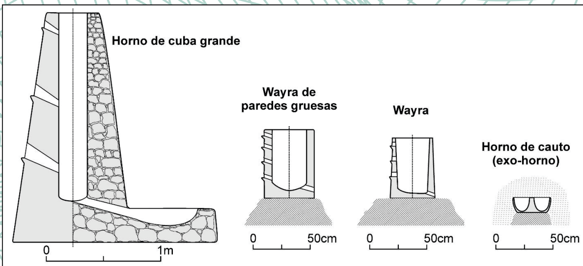
Figura 4 Modelos de hornos metalúrgicos prehispánicos identificados en Cobres.
